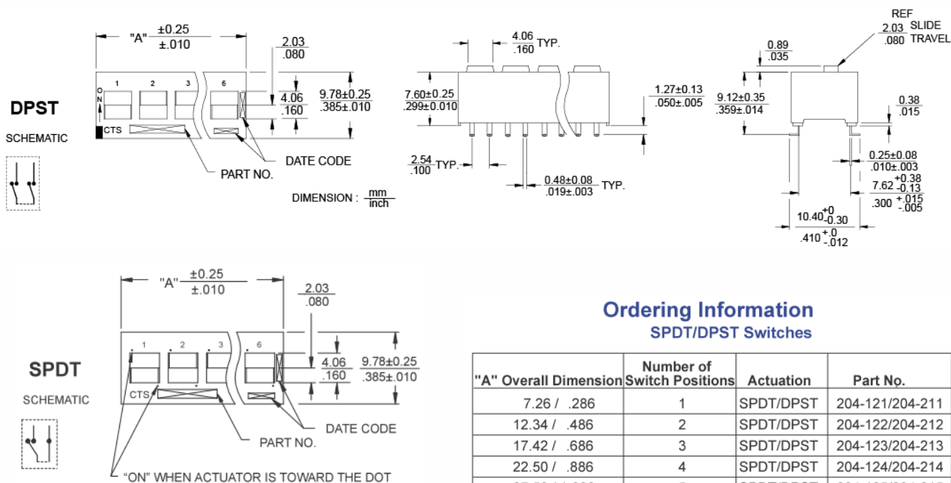
Figure 2 – SPDT/DPST
